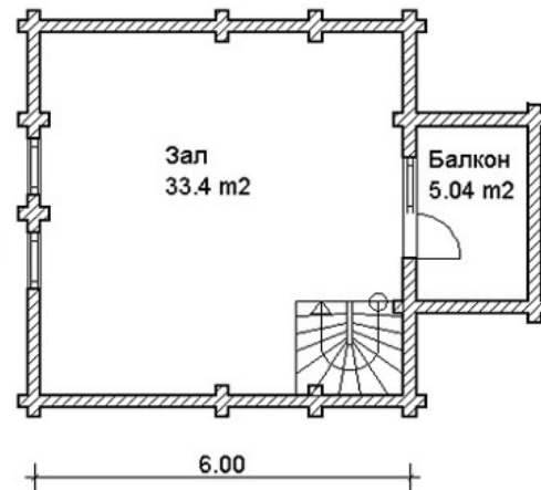
План мансарды
