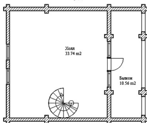
План мансарды
