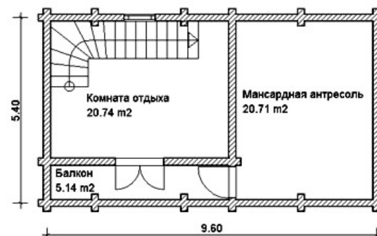
План мансарды
