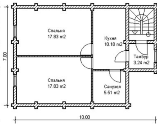
ПЛАН МАНСАРДЫ
