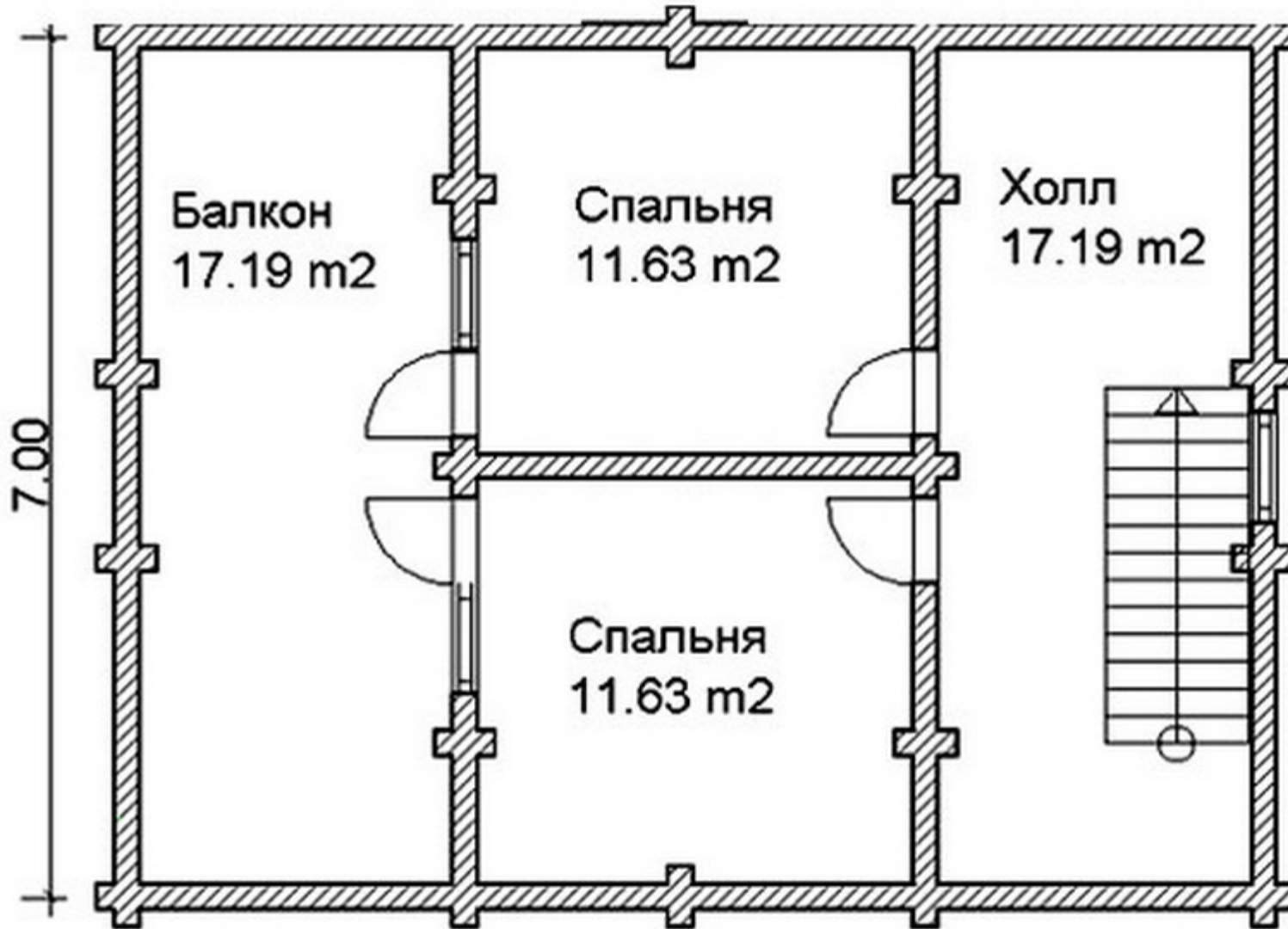
ПЛАН МАНСАРДЫ
