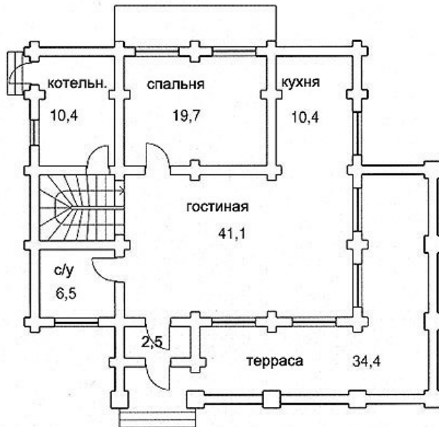
План 1 этажа
