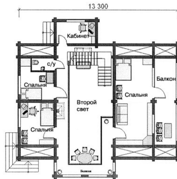
ПЛАН МАНСАРДЫ
