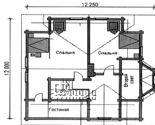
План 2 этажа
