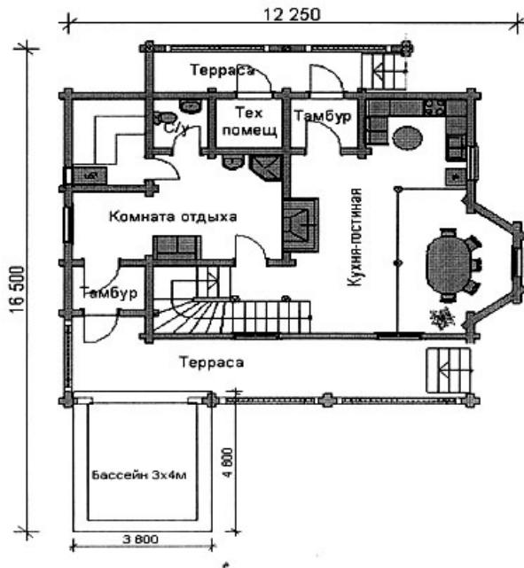
План 1 этажа
